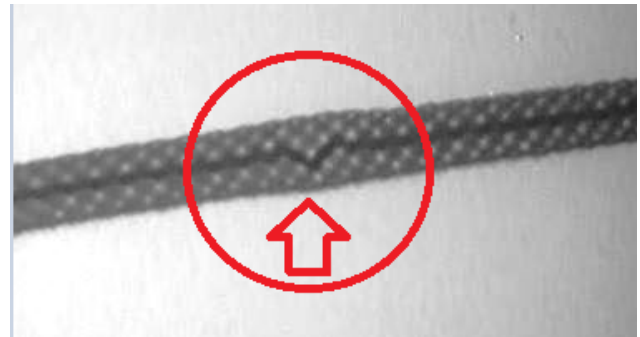
Recherche de défauts de connexion ou de points chauds des fils chauffants par rayons X (écran de protection enlevé pour la prise de vue). Exemple de point chaud détecté : épaisseur entre les conducteurs chauffants.
