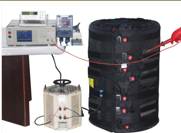
Dispositif d'essai de mesure du courant de fuite à chaud
