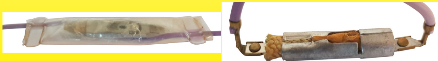
Limiteur de température de couverture chauffante, à rupture lente, utilisé conjointement avec un système de régulation de puissance anglais GEC (General Electric Company). Il est recouvert d'un manchon PVC étanche soudé sur les fils. Vers 1970 (Collection Ultimheat)
