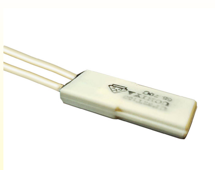
1980 ca Limiteur bimétallique étanche Uchiya UP32 sur couverture chauffante de la marque de distributeur Gitem. (Collection Ultimheat)
